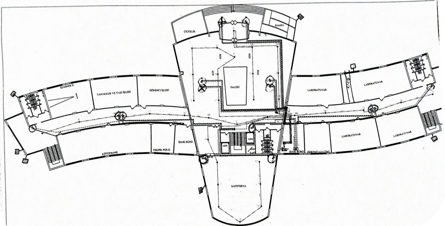
VAKLE MYD ZEMİN KAT PLANI
